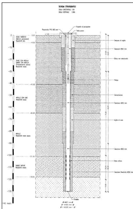
Progetto del nuovo pozzo
